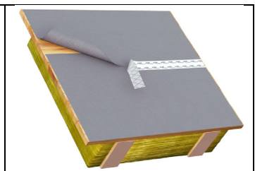
Abb. 6: Überlappung außen
