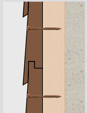
Sichtbare Verschraubung
