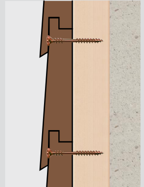
Nicht sichtbare Verschraubung
