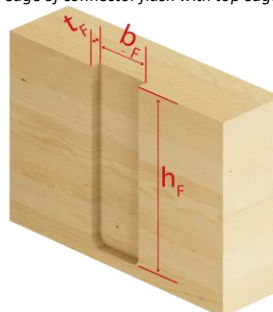
Im Hauptträger eingelassen Embedded in header
