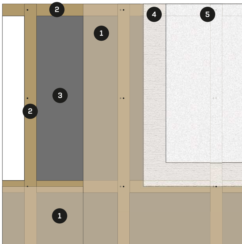
istraw-Wandssystem – Masstab 1:20
